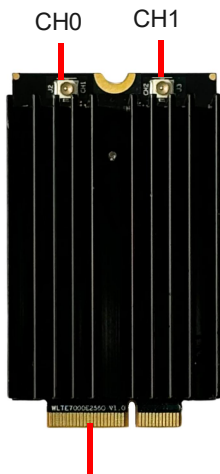
M.2 E Key Edge Connector
